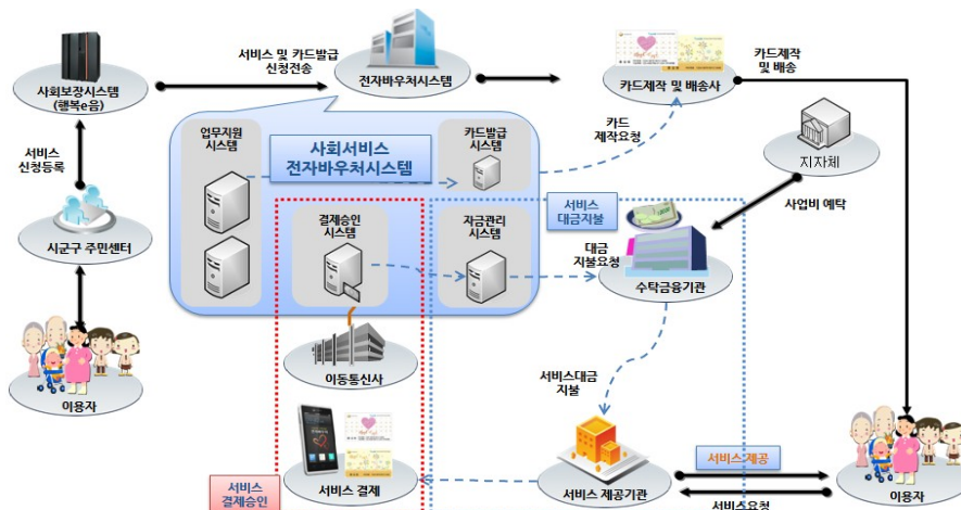
■ 전자바우처 운영흐름도 ■
